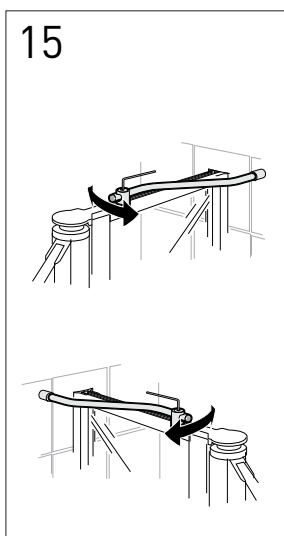
Justera sidoglasets i sidled genom att först lätta på skruven i stagets överkant, justera därefter sidoglas och till sist drag åt skruven igen.
