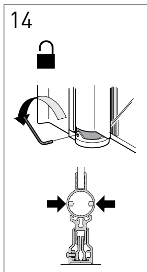
Lås upp positionsbrickans låsskruvar och ställ dörrarna i ett läge där dörrbladets magnetlist möter det sidoglasets. Om magnetlisterna ej möts justeras sidoglasens position enligt bild 15.
