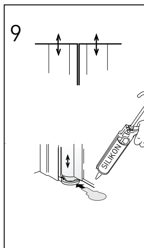
Dörrbladens överkant skall linjera. Justera vid behov genom att använda de gitarrformade distansklossarna. Applicera Superfix mellan golv och golvbeslag. Används distansklossar skall Superfix även appliceras på dessa.
