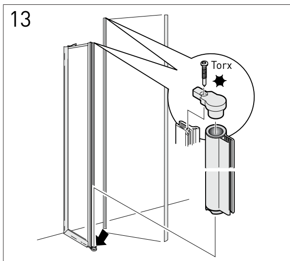
Montera de båda dörrbladen. Observera att dörrbladen skall sättas i rakt ovanifrån på sidoglasets nedre gångjärnsbeslag. Lås därefter dörrbladen i överkant genom att skruva fast sido-glasets övre gångjärnsbeslag.
