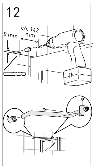
Montera sidoglasens stag. Applicera Superfix / våtrumssilikon i borrhålen.
