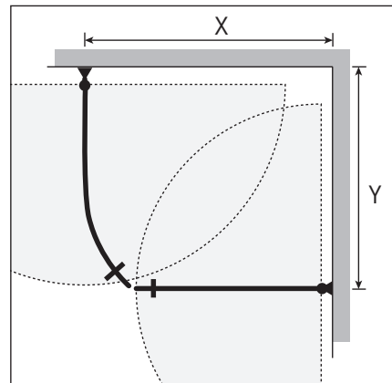
Vänsterhängd dörr
