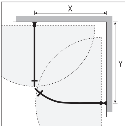
Högerhängd dörr
