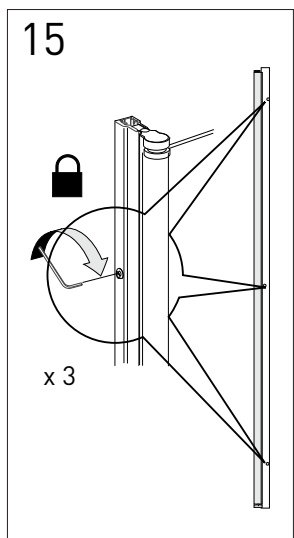
Lås dörrbladet vid väggprofilen med väggprofilens tre spännskruvar. Spännskruvarna skall efterdras efter ca 14 dagars användning.
