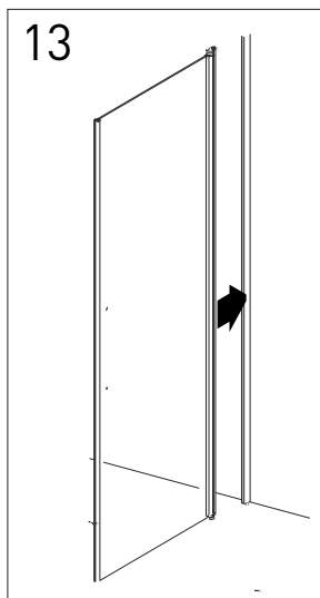
Tryck fast dörrbladet i väggprofilen. Säkerställ att dörren är rättvänd.
