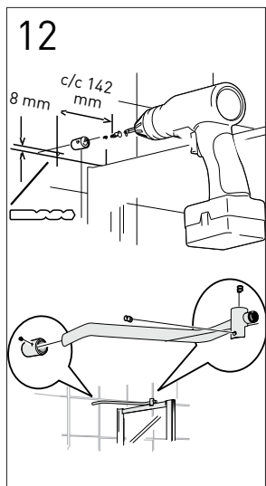
Montera sidoglasens stag. Applicera silikon i borrhålen.
