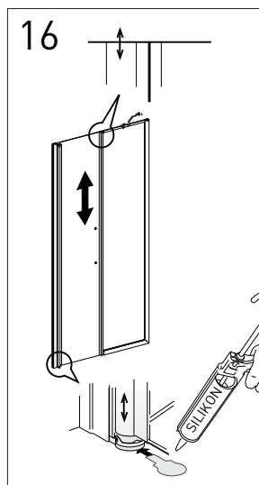
Dörrbladens överkant skall linjera. Justera vid behov genom att använda de gitarrformade distansklossarna. Applicera silikon mellan golvet och golvbeslag. Används distansklossar skall silikon även appliceras på dessa.
