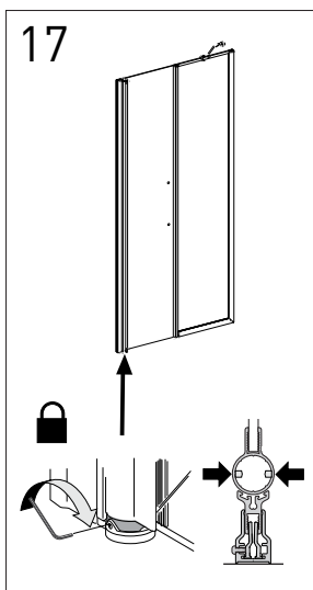
Dörrens stängningsläge bestäms av positionsbrickan. Lås positionsbrickan med dess två låsskruvar i önskat läge.
