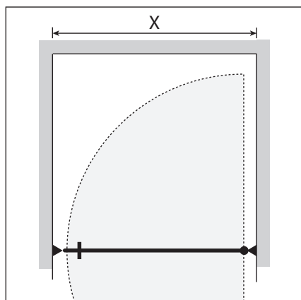
Högerhängd dörr
